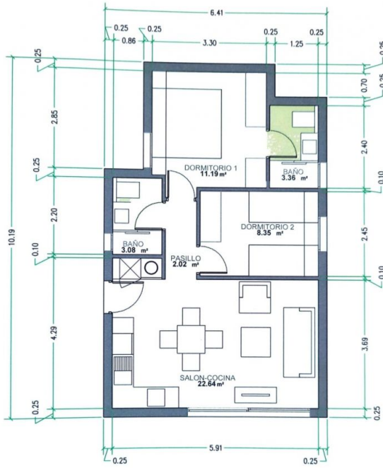
TIPO VIVIENDA PLANTA BAJA.
