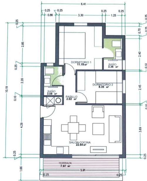
TIPO VIVIENDA PLANTA ALTA. CONSTRUIDA. 60.44 m 2 UTIL TOTAL. 50.64 m 2
