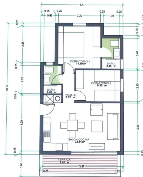
TIPO VIVIENDA PLANTA ALTA. CONSTRUIDA. 60.44 m² UTIL TOTAL. 50.64 m²
